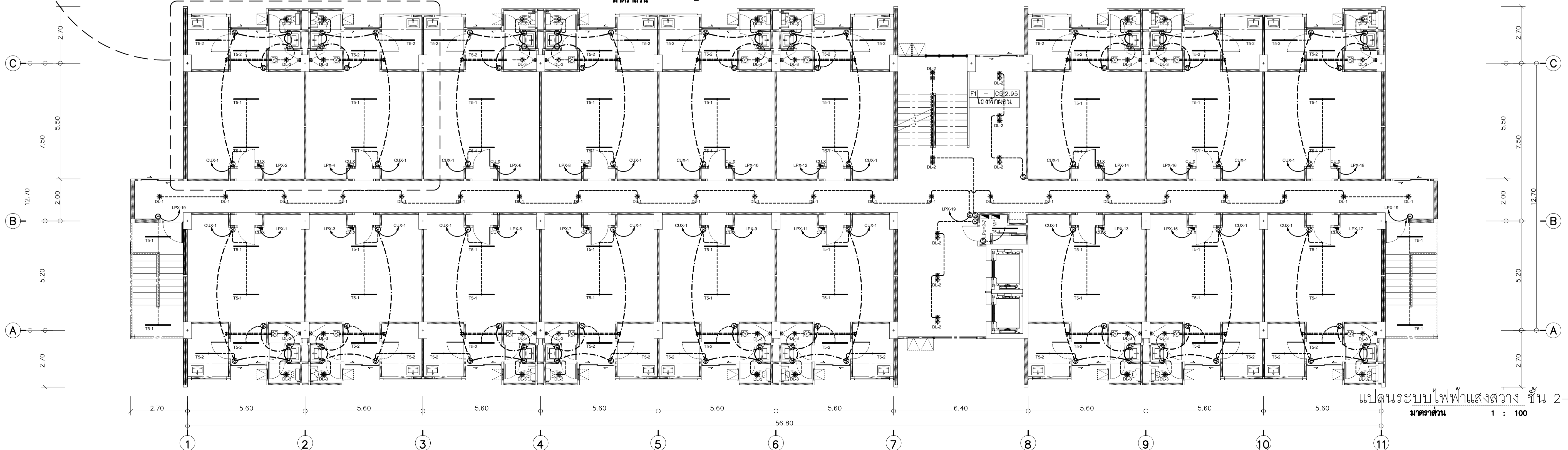
แปลนขยายตำแหน่งติดตั้งหลอดอากาศ ห้องพัก มาตราส่วน
