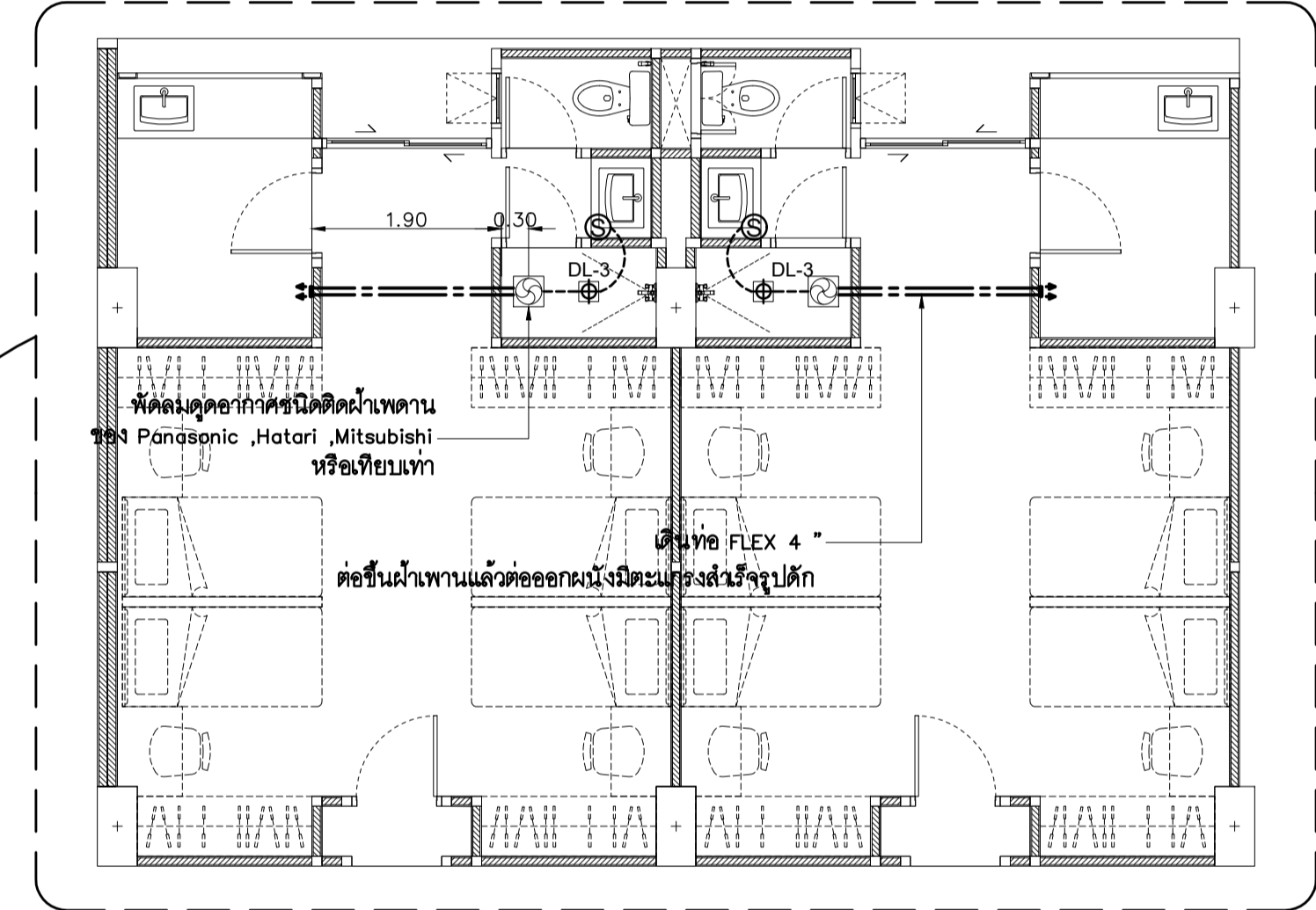
แปลนขยายตำแหน่งติดตั้งหลอดอากาศ ห้องพัก มาตราส่วน
