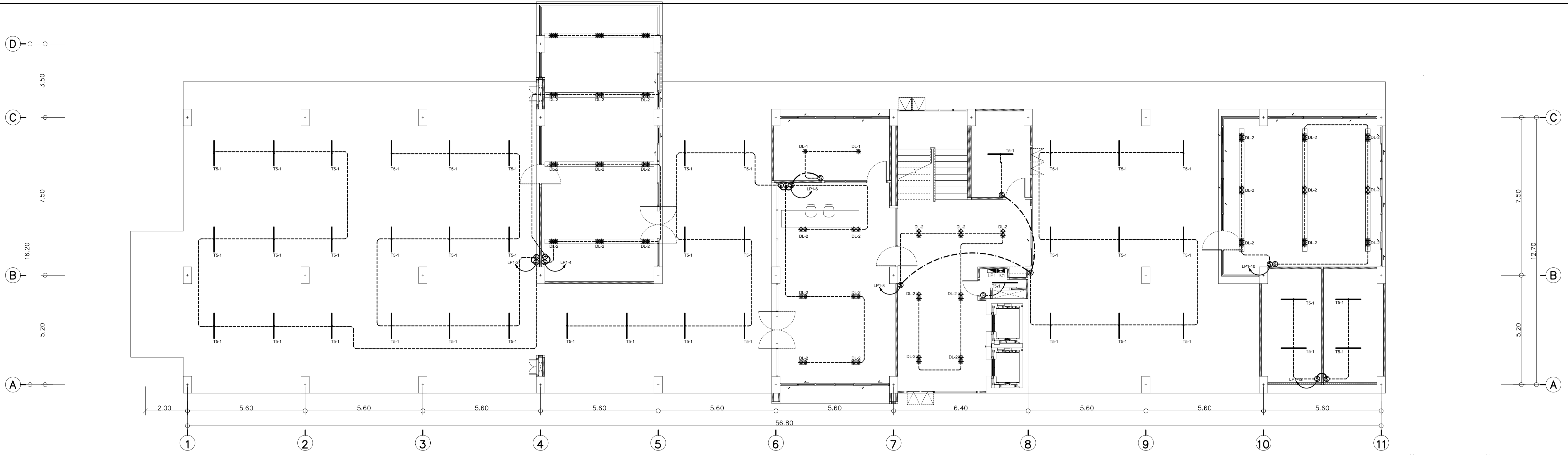
แปลนระบบไฟฟ้าแสงสว่าง ชั้น 1 มาตราส่วน 1 : 100
