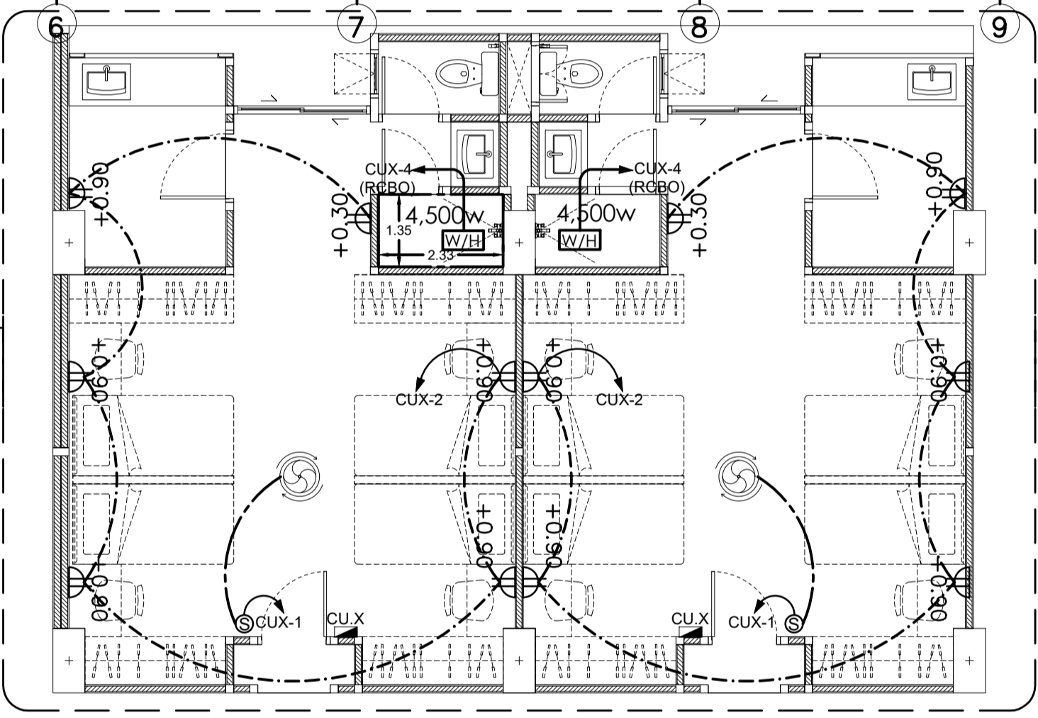
แปลนระบบ PLUG & TELEPHONE & LAN ชั้นที่ 1 มาตราส่วน 1 : 100
