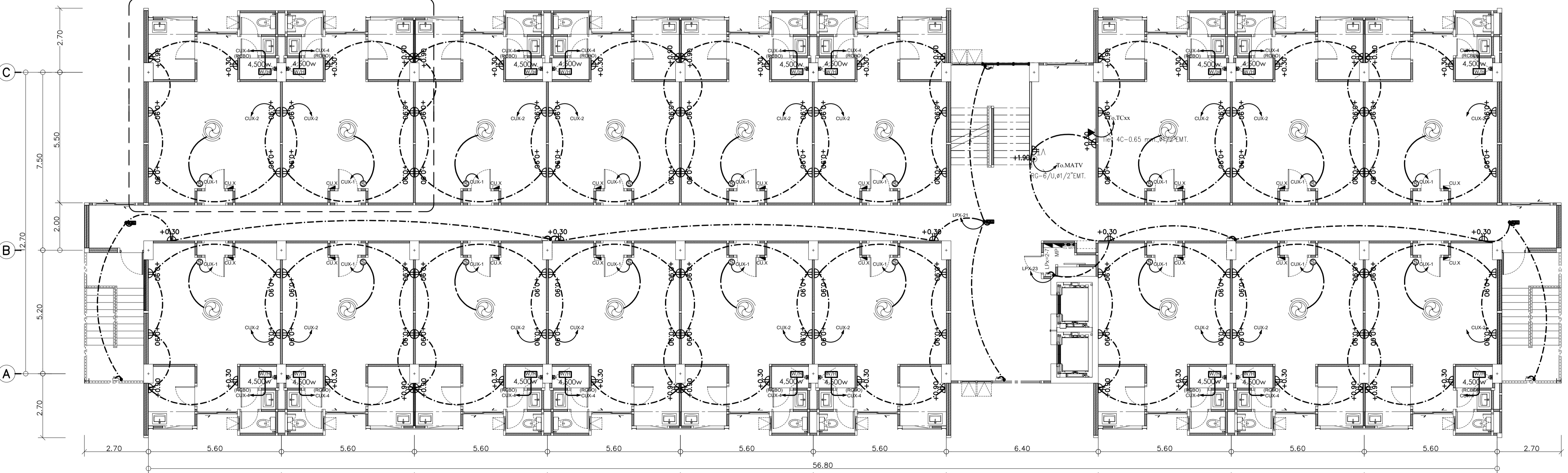
แปลนระบบ PLUG & TELEPHONE & LAN ชั้นที่ 2-7 มาตราส่วน 1 : 100
